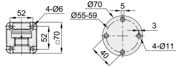
底座安装尺寸(共用)
