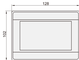
A向视图
