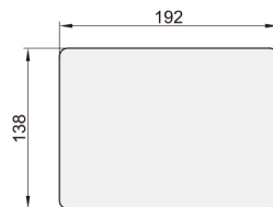
■开孔尺寸图
