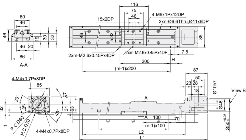
■ 不含护盖尺寸图
