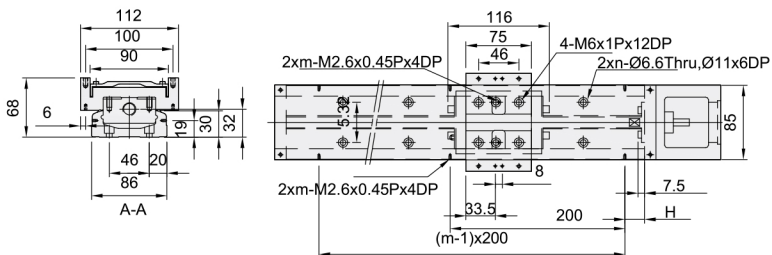
■ 含护盖尺寸图
