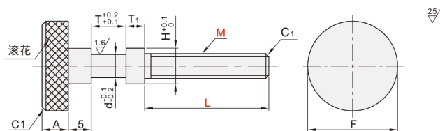
滚花旋钮型 YAZ31 YAZ32 YAZ33
