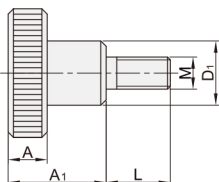
带台阶 外螺纹型 SJA81
