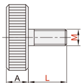
无台阶 外螺纹型 SJA61
