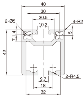
XCS01-4042HL
