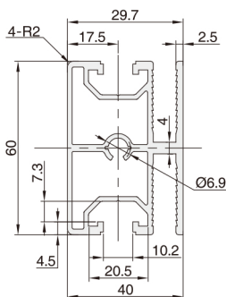
XCS01-4060HL
