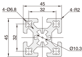
XCS01-4545Y
