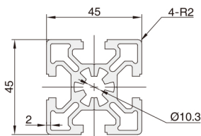
XCS01-4545E
