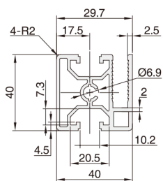
XCS01-4040HL
