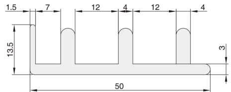
XCPE01-T
