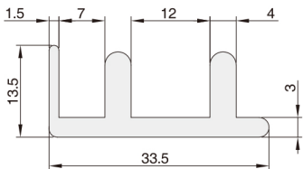
XCPE01-E
