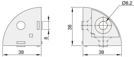
XCCN56-408-H (三维连接件)
