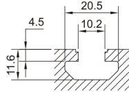
槽口详图
