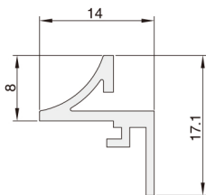
XCPB01-308-1417 (后装面板座)
