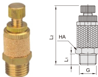
DCG31-BSLE-G B型排气节消声器
