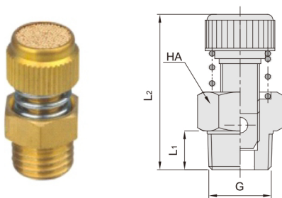
DCG21-SD-G 调速消声器
