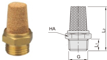
DCG01-SL 通用消声器
