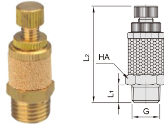
DCG31-BSLE-G B型排气节消声器
