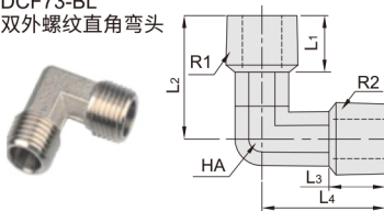
DCF73-BL 双外螺纹直角弯头
