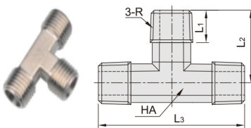
DCF61-BT 内外螺纹三通
