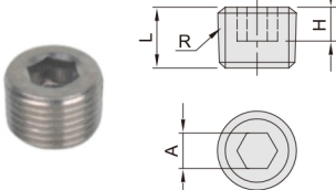
DCF41-BP 内六角堵头
