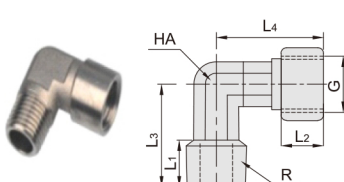
DCF71-BLM 内外螺纹弯头
