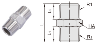
DCF11-BB 双外螺纹直通
