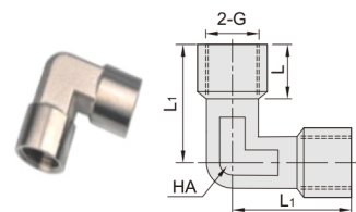
DCF72-BLF 双内螺纹直角弯头
