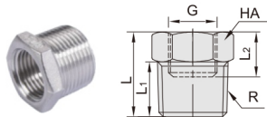
DCF31-BD 内外螺纹直通
