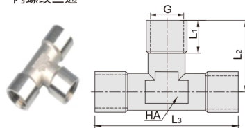
DCF51-BF 内螺纹三通
