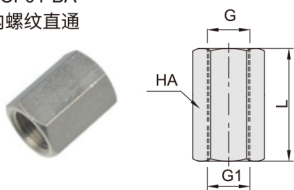
DCF01-BA 内螺纹直通
