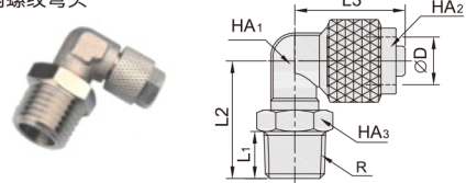
DCE12-CBL 快拧内螺纹弯头
