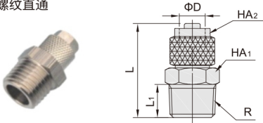
DCE13-CBC 快拧螺纹直通
