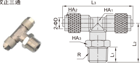
DCE14-CBT 快拧螺纹正三通
