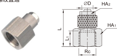
DCE11-CBF 快拧内螺纹直通
