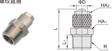
DCE13-CBC 快拧螺纹直通
