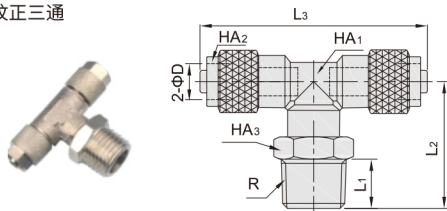
DCE14-CBT 快拧螺纹正三通
