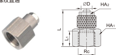
DCE11-CBF 快拧内螺纹直通
