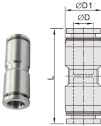
DCC51-SSU 联管直通
