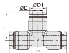
DCC31-SSE 联管正三通
