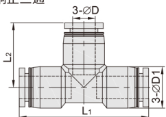
DCD07-BPE 全铜正三通
