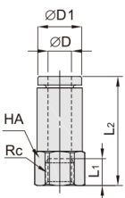
DCD01-BPCF 全铜内螺纹直通
