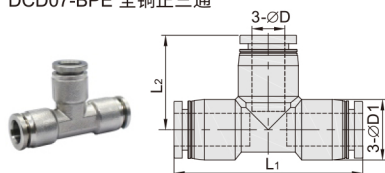
DCD07-BPE 全铜正三通
