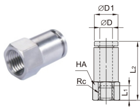
DCD01-BPCF 全铜内螺纹直通
