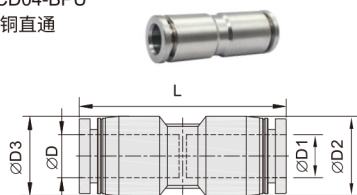
DCD04-BPU 全铜直通
