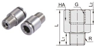
DCB61-CPCVC 单向阀
