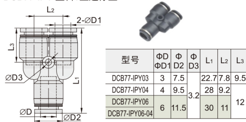
DCB77-IPY 塑料Y型迷你型
