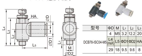
DCB78-ISC04 迷你节流阀
