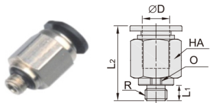
DCB71-IPC 螺纹直通迷你型
