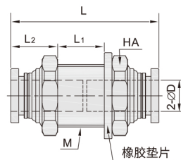
DCA81-CPM 隔板直通
