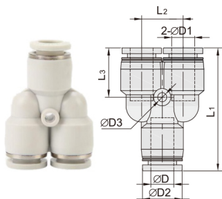
DCA72-CPY 塑料Y三通
