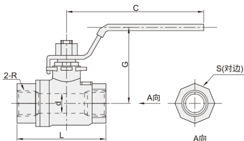
全铜球阀 DCW51
