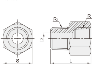
管套型 内外螺纹 DCN06
