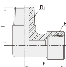
弯管型 内外螺纹 DCN16
