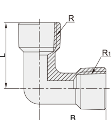
弯管型 内螺纹 DCN21
