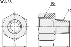
异径内外螺纹套管 DCN36
