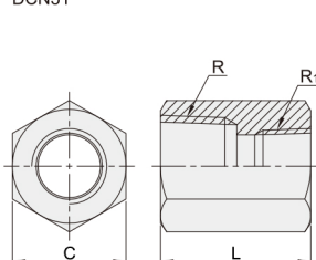
异径六角套管 内螺纹 DCN31
