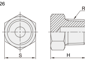
管塞型 外螺纹 DCN26
