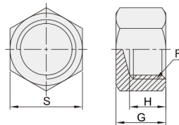
盖型 DCN11
