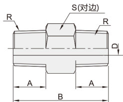
直接头 外螺纹同径 DCM51
