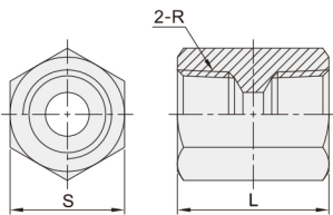
管套型 DCN01
