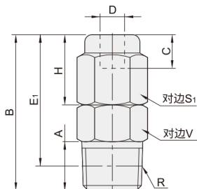
直接头/外螺纹 DCY01
