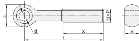
活节螺栓 YAH03
