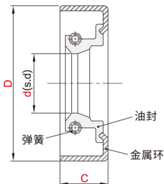
单唇型 外周金属型 YXE12
