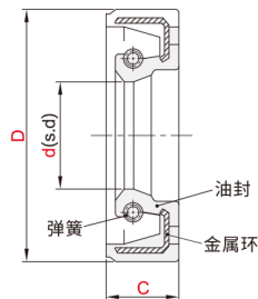
外周橡胶型 YXE13
