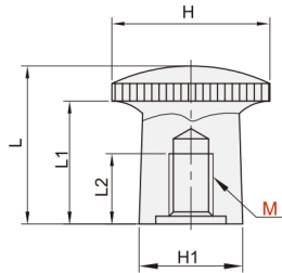
带锁紧螺帽 YZB11/YZB12
