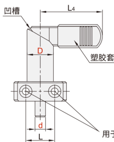
带塑胶套 YZU42
