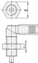
带锁紧螺帽 YZU33/YZU34
