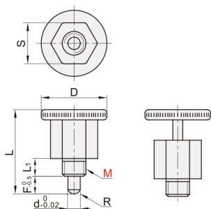
复位型 YZU01/YZU02
