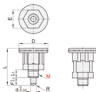
自锁型 YZU11/YZU12
