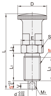
无锁紧螺帽 YZT11/YZT12
