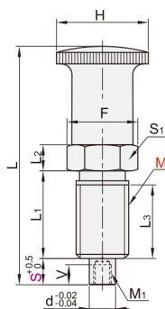
无锁紧螺帽 YZT01/YZT02
