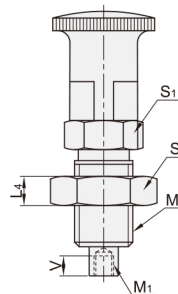
带锁紧螺帽 YZT13/YZT14
