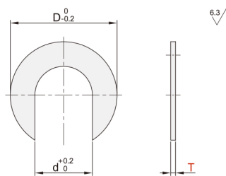
开口型 YEC01/02
