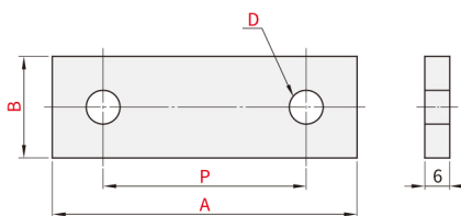
双孔型 YWJ31/32/33
