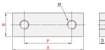
双螺孔型 YWJ11/12/13
