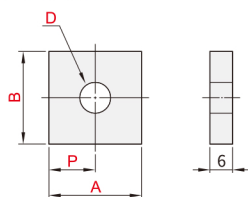
单孔型 YWJ21/22/23
