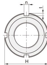
圆螺母 YBP02/03
