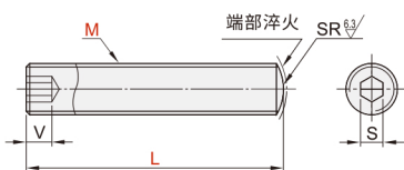
内六角孔型
