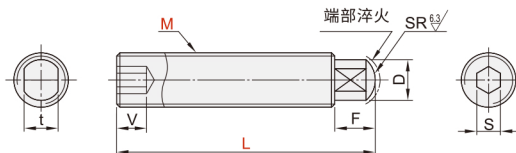
内六角孔带扳手槽型
