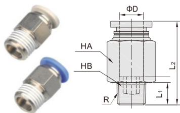
DCA01-CPC螺纹直通
