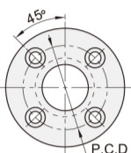
安装法兰 圆法兰型
