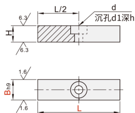
B型 PLF41/42
