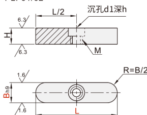
中心螺纹沉孔型 A型 PLF61/62
