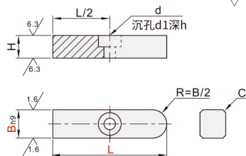
C型 PLF51/52
