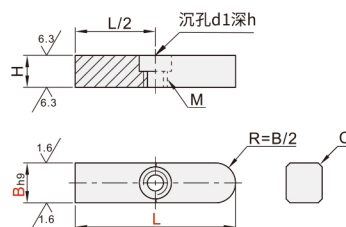
C型 PLF81/82
