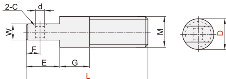
带扁方半牙型 AFD01 AFD11
