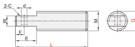
带扁方全牙型 AFN01 AFN11
