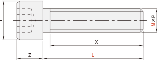
内六角圆柱头螺钉 YAB01/02/03
