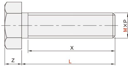
外六角头螺栓 YAB11/12
