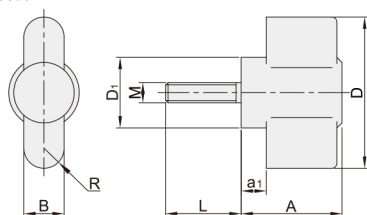
外螺纹型 SJA41
