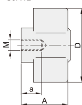
内螺纹型 SJA42
