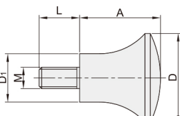
外螺纹型 SJA32
