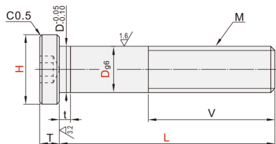
L尺寸选择型 BTP01/02/06
