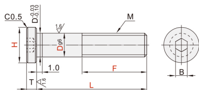
螺栓型 BTP21/BTP22/BTP27
