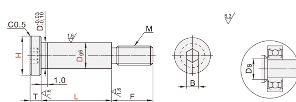
肩型 BTP31/BTP32/BTP37
