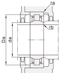
(安装图)
