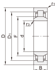
外圈无挡边 BDN11
