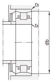
(安装图)
