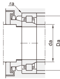
(安装图)
