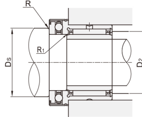
(安装图)
