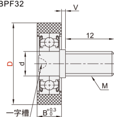
长螺纹型 BPF32
