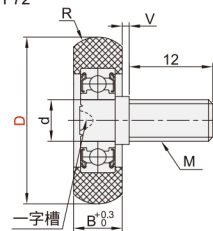
长螺纹型 BPF72
