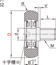
外螺纹型 BPF51 BPF52
