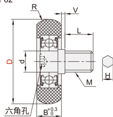
内六角外螺纹型 BPF62
