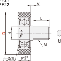
内六角外螺纹型 BPF21 BPF22
