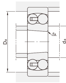
(安装图)
