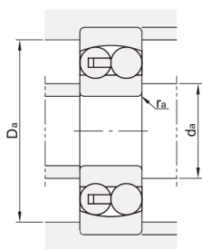
(安装图)
