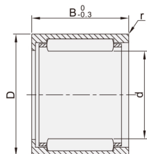
开式 BHK01 BHKJ01
